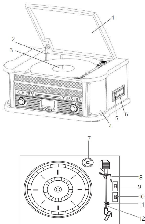
Tourne-disques
